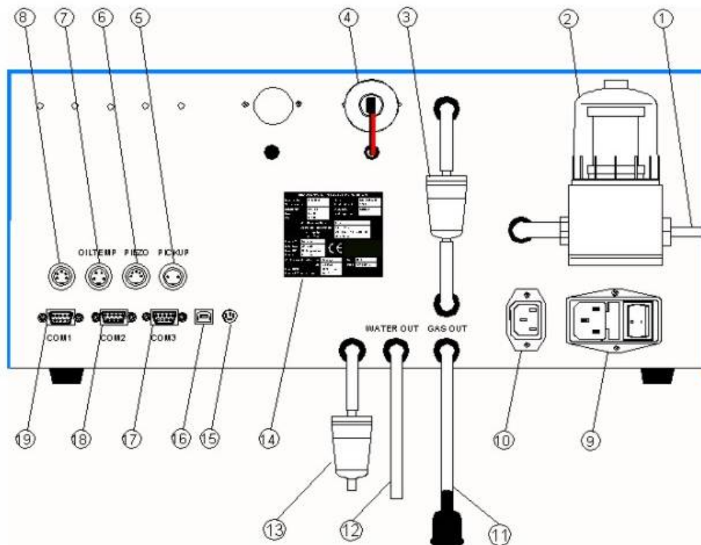
Figuur 2. Achterzijde van de VLT-E8104
