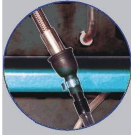
Figuur 14. Verbinden van de lektestadapter
