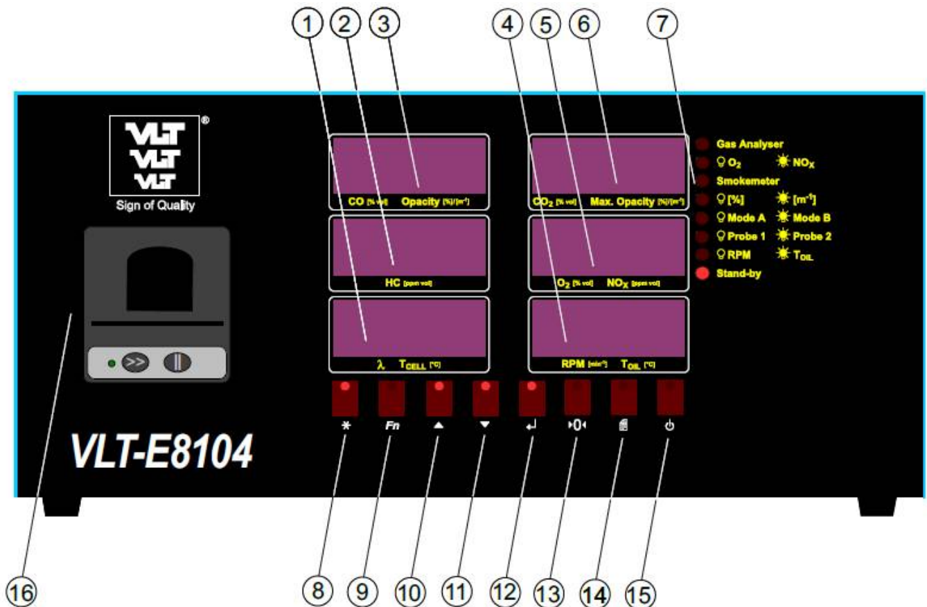
Figuur 1. Voorzijde van de VLT-E8104
